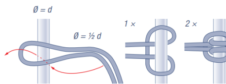
Doppelter Spierenstich (z.B. für Prusikschlinge)
